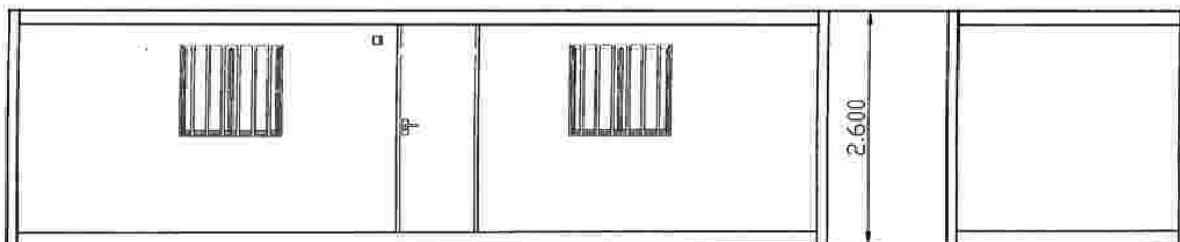
2 Bureaus + wc 2 Oficinas + Aseo 2 Offices with wc 8.200 x 2.400 mm
