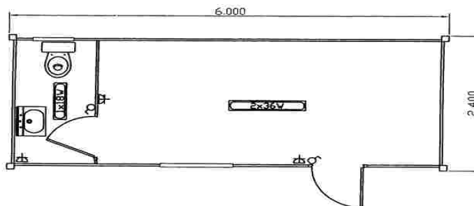
Bureau avec wc Oficina + Aseo Office with wc 6.000 x 2.400 mm
